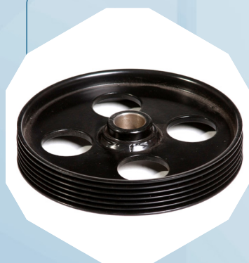
پولی پمپ هیدرولیک پژو ۴۰۵ Peugeot 405 Hydraulic pump pulley
